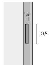
maniglia incassata inset handle
