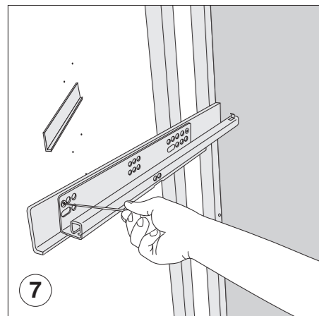
Avvitare le piastre al montante (fig. 4-5) e riavvitare le guide alle piastre (fig. 6-7). Screw-up the plates to the upright (fig. 4-5) and rescrew-up guides to the plates (fig. 6-7).
