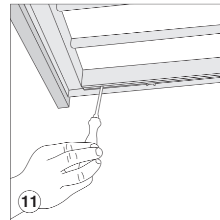
Estrarre le guide (fig. 8), inserire l'elemento estraibile, mantenendolo inclinato (fig. 9-10). Fissare lo stesso alle guide (fig. 11) per mezzo delle viti in dotazione. Remove the guides (fig. 8) insert the removable element keeping it inclined (fig. 9-10). Fix it to the guides (fig. 11) using the supplied screws.
