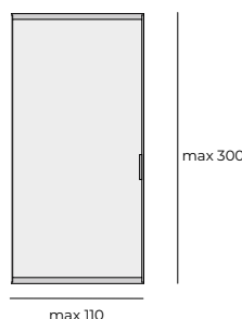
Anta per sistema basculante Pivot door
